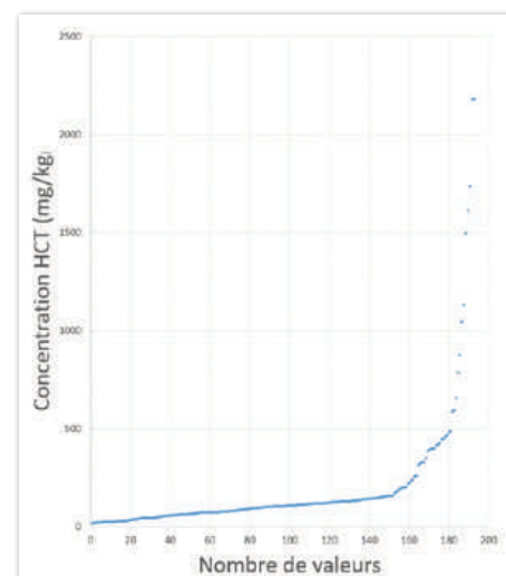
Répartition des concentrations en hydrocarbures totaux dans les sols (site confidentiel)
